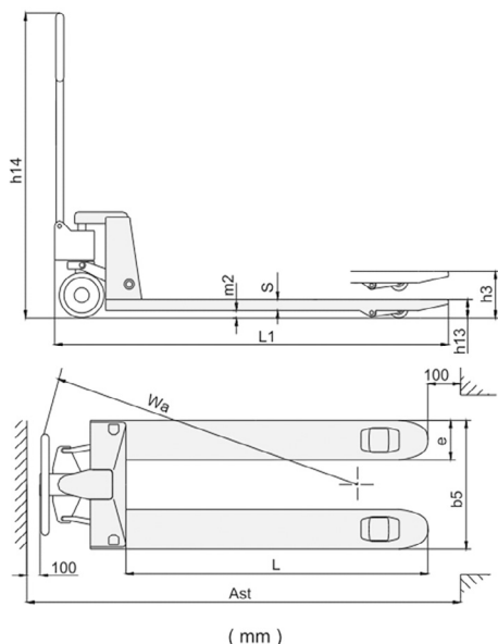
Fig. 1 – Relação de dimensões
