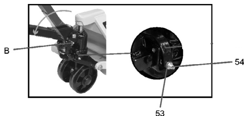
Fig. 6 – Retirando el pasador
